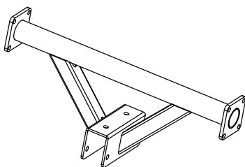
Grupo de soldagem fixa de placa de sino
